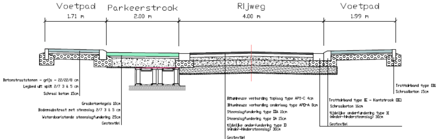
Typedwarsprofiel 5
