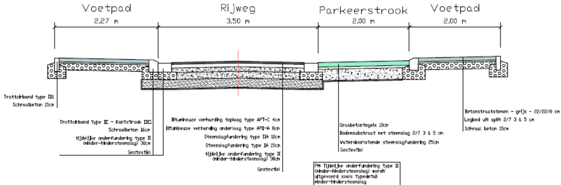
Typedwarsprofiel 1
