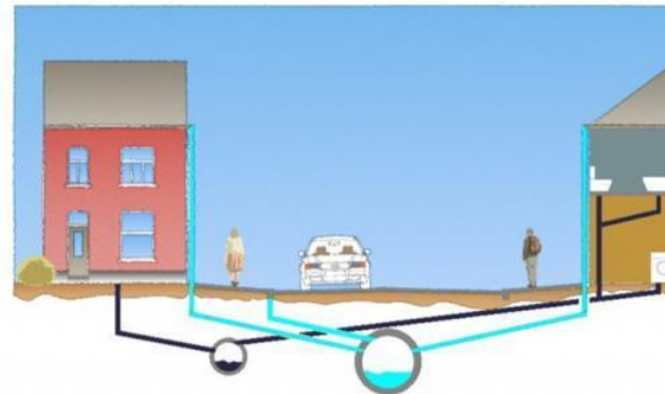
Gescheiden stelsel
