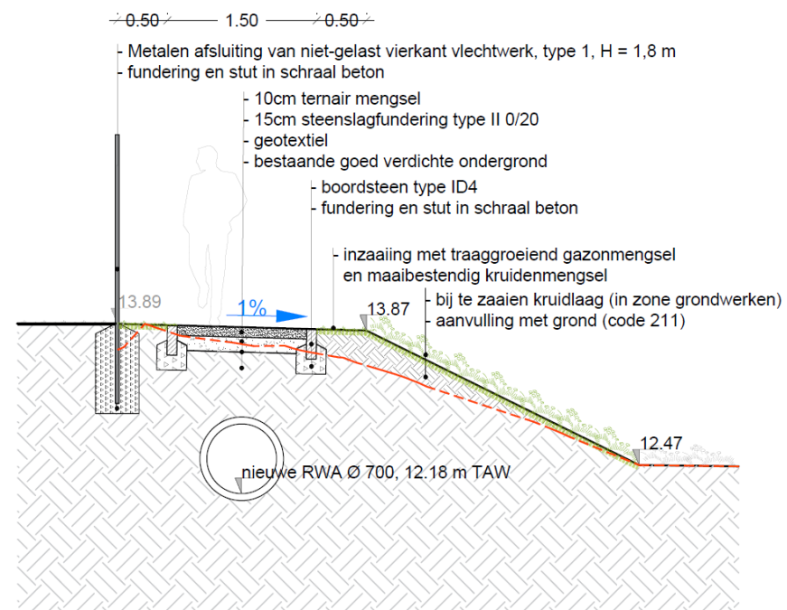
Profiel PRD 1 - Kruiwagenpad in halfverharding Schaal 1/50
